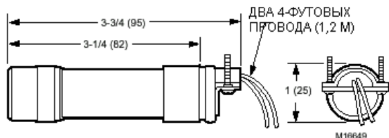
Рисунок 4. Установочные размеры C7927A1016 (версия для США) в дюймах (мм)
